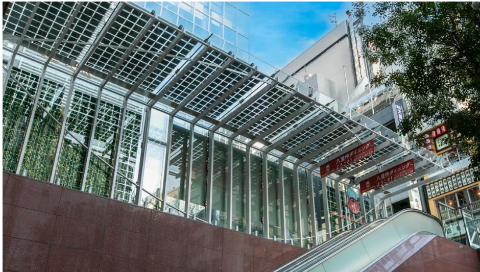
東京建物八重洲ビル ステップテラスに導入された AGC の太陽光発電ガラス サンジュール®
